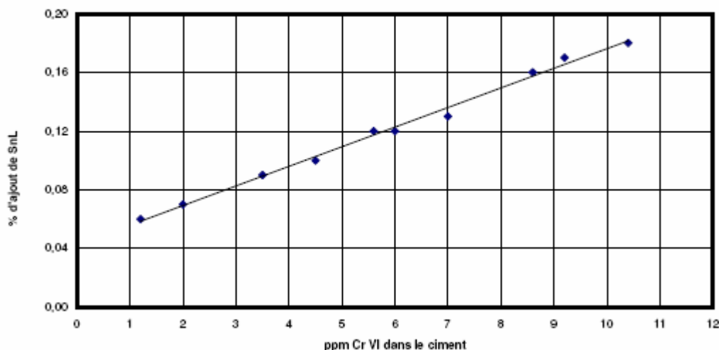
Principe de dosage
